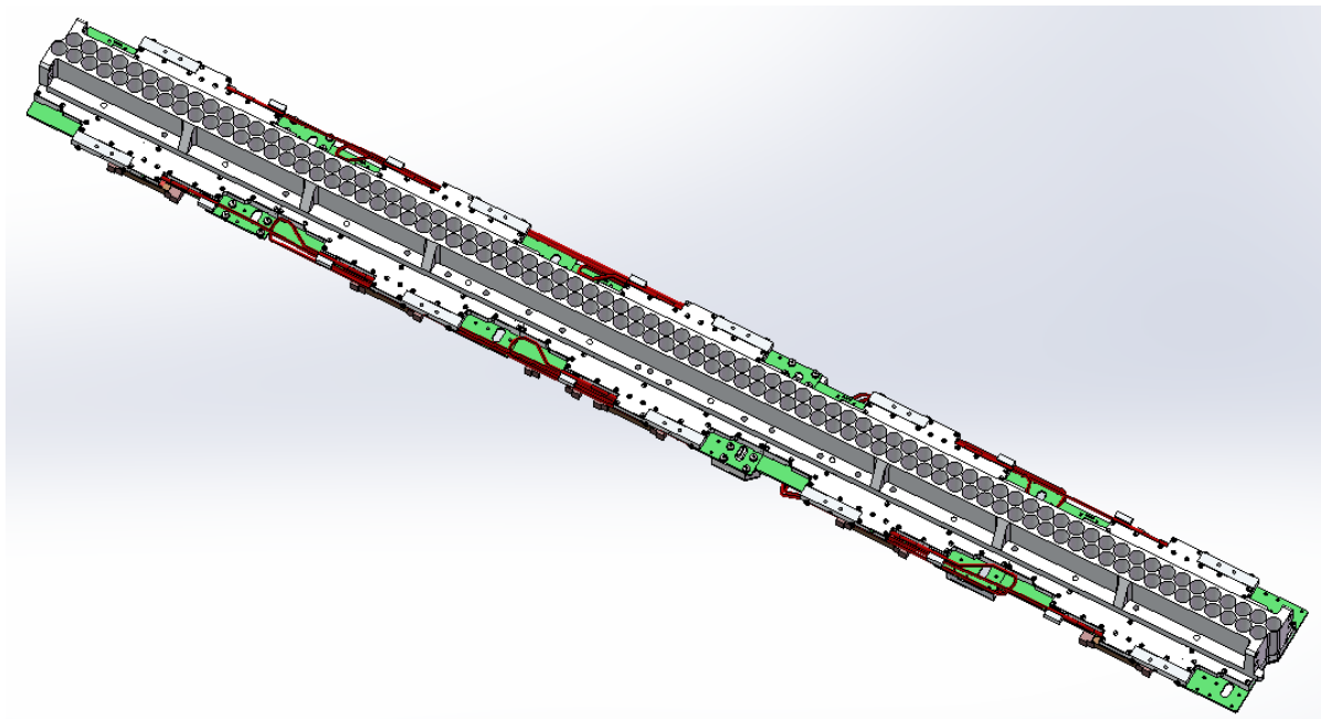
收发 80 路开关装上天线示意图
