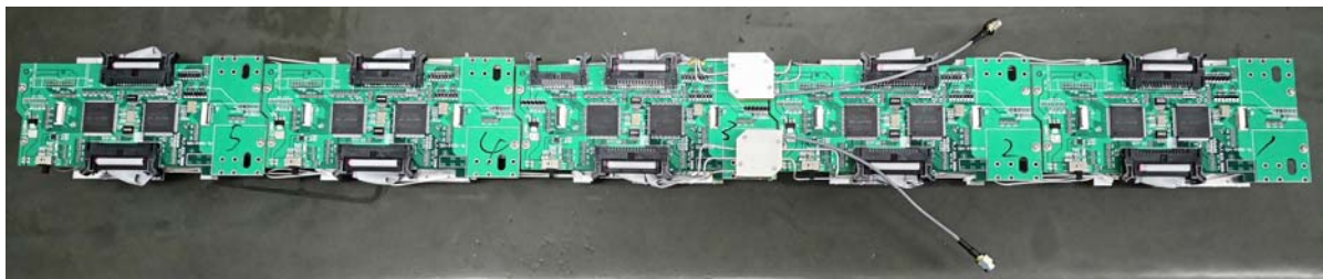
收发 80 路开关组件背面图
